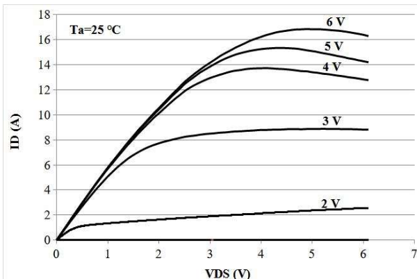
I_{DS} vs. V_{DS} @ T_j = 25^\circ\text{C}
