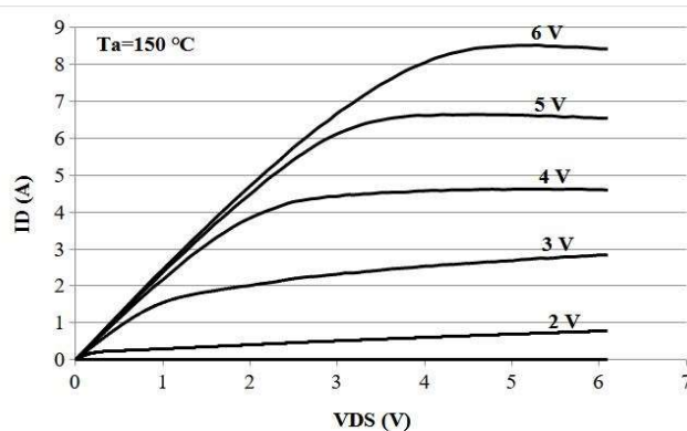
I_{DS} vs. V_{DS} @ T_j = 150^\circ\text{C}
