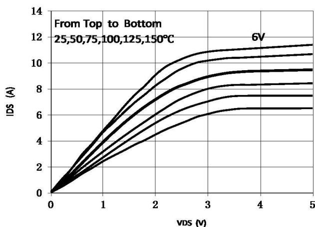
I_{DS} vs. V_{DS} @ V_{GS} = 6\text{V} , T_j = 25-150^\circ\text{C}
